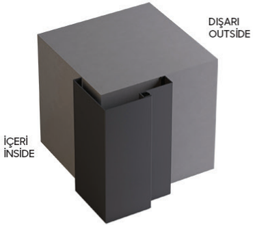
Dışardan Geçme Kasa (Fransız Tipi) External Mounted Fixed Frame (French Type)
