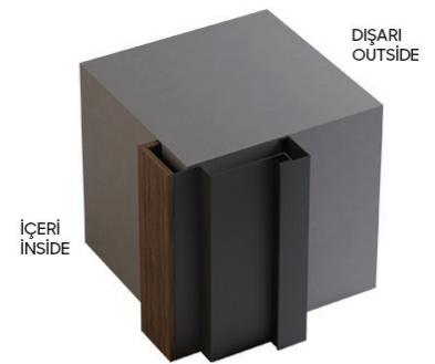
Dışardan Geçme Dışa Açılır Kaplamalı Kasa (Rus Tipi) External Mounted Fixed Covered Frame-Opening Outwards (Russian Type)
