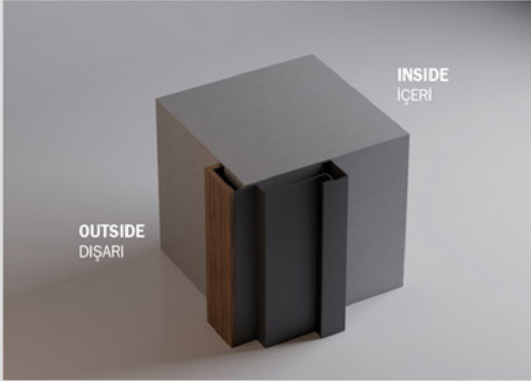
External Mounted Fixed Covered Frame-Opening Outwards (Russian Type) Dışardan Geçme Dışa Açılır Kaplamalı Kasa (Rus Tipi)
