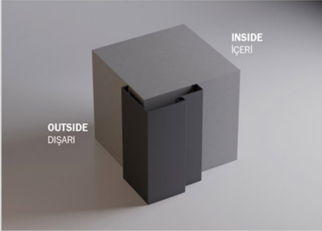
External Mounted Fixed Frame (Standard Type) Dışardan Geçme Kasa (Açık Tipi)
